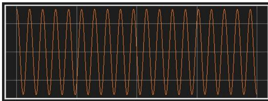
Figura 1. Esta gráfica corresponde a una nota musical. Es decir, un sonido limpio y sostenido en el tiempo, con una frecuencia fija. El tubo está sonando en su frecuencia de resonancia.
